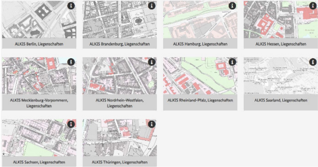
Şekil 9. Geoportal’da Ekim 2021 itibariyle erişime açık, eyalet seviyesinde kadastral veri setleri. 16 eyaletin yalnızca 10 adedinin veri setinin erişime açık olduğu görülmektedir.
